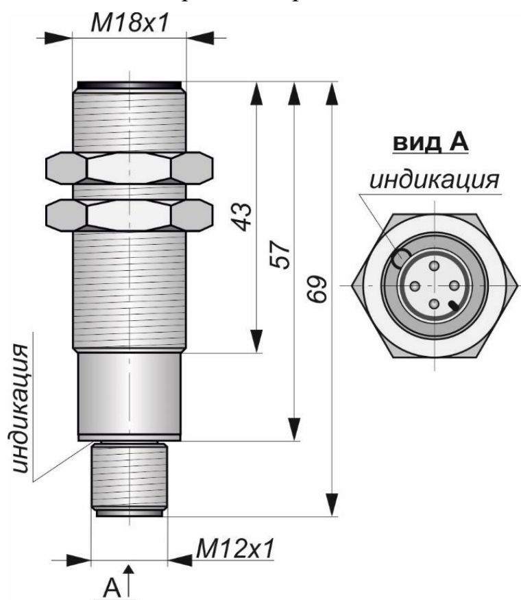
Габаритный чертеж
